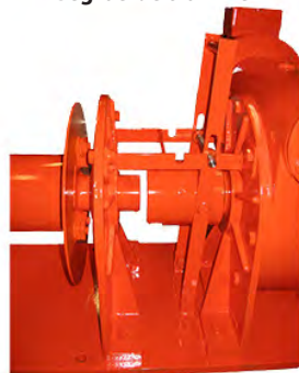
Vrijloopp koppeling
